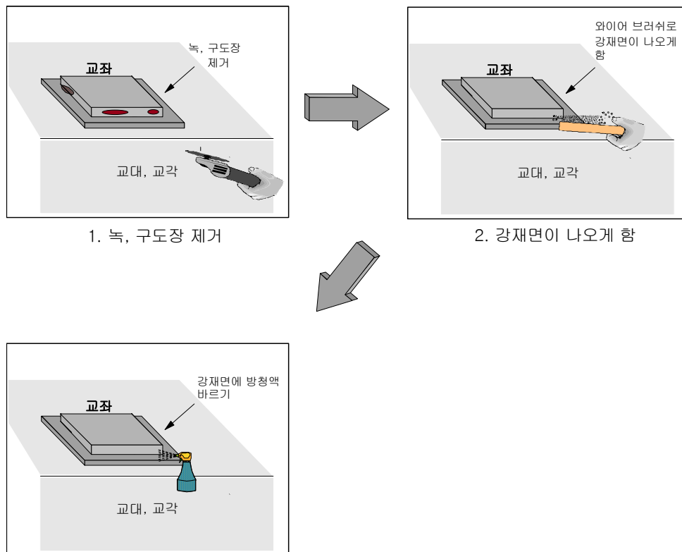
<그림 6.3.9> 교량반침 방청순서도
